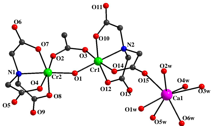
Fig. 1. Structura compusului trinuclear [CaCr_2(?-OH)(?-OAc)(nta)_2 \cdot 6H_2O] \cdot 2H_2O .
