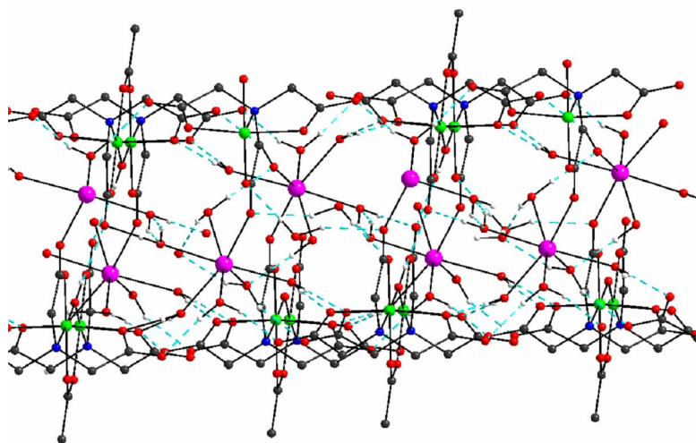
Fig. 2. Stratul 2D in structura compusului [CaCr_2(?-OH)(?-OAc)(nta)_2 \cdot 6H_2O] \cdot 2H_2O (atomii de hidrogen ce nu fac parte din legăturile de hidrogen sunt omise pentru claritate)
